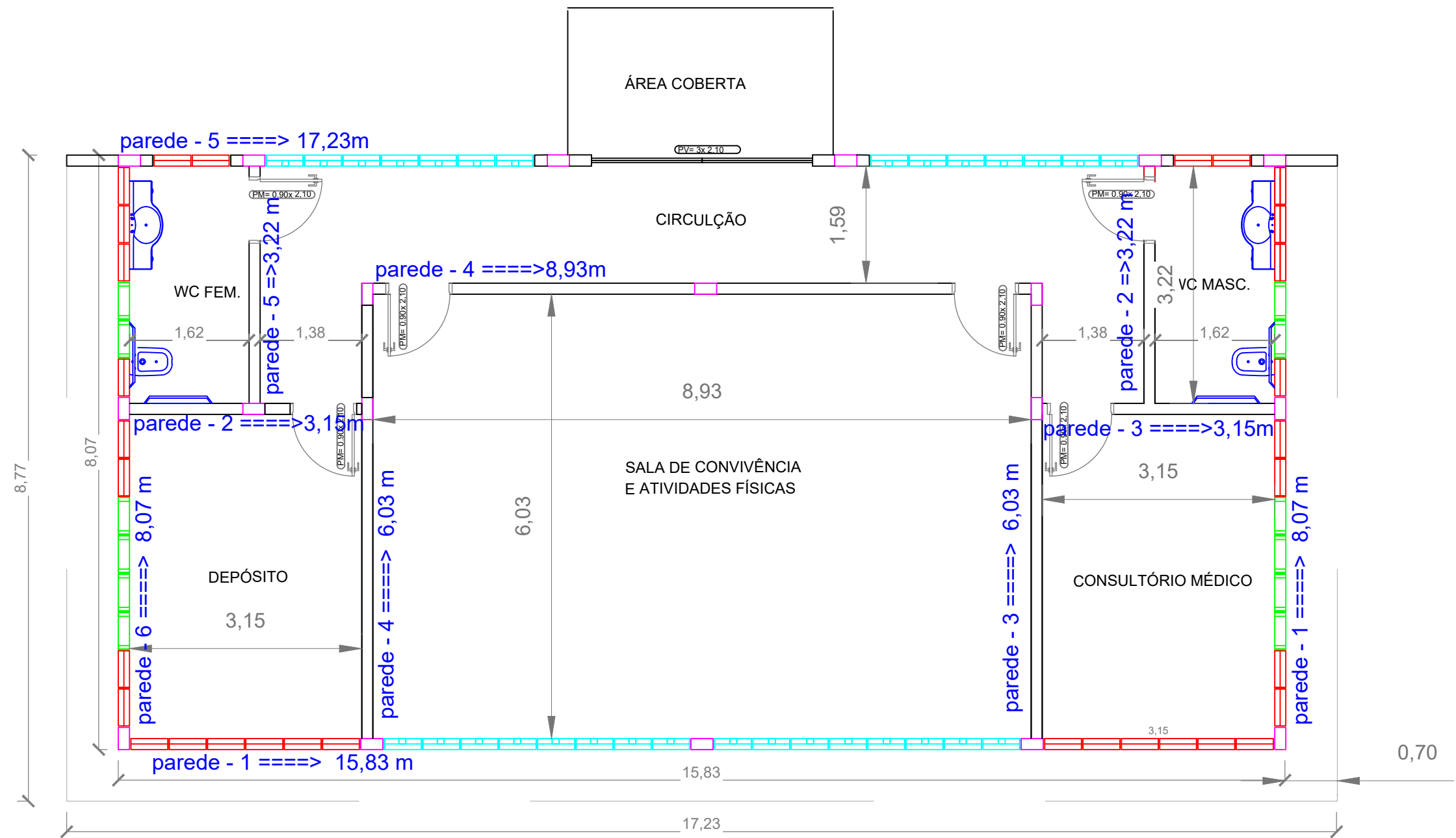
PLANTA BAIXA ESCALA : 1/75
